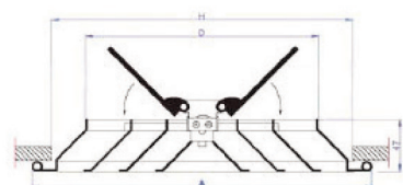
Diffuseur Dimensions (mm)
