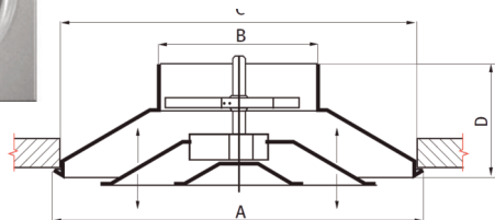
Diffuseur Dimensions (mm)
